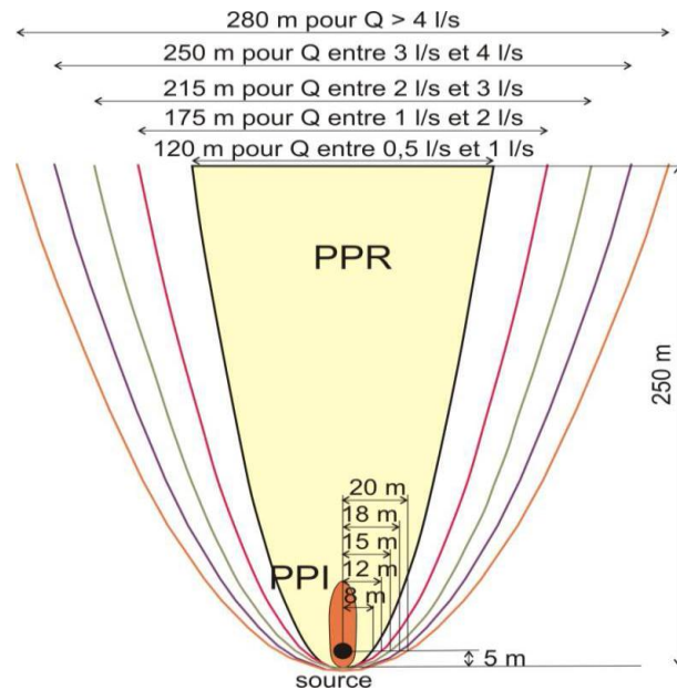
Figure I.7 : Périmètre de protection rapproché d'une source (Vassolo 2014).
