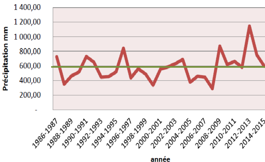
Figure II.5: Variation des précipitations annuelles au niveau de la station de Mefrouche (1986-2015) (DRE Tlemcen, 2015)
