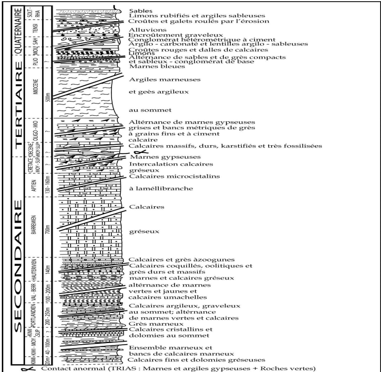
Figure I.6: Log lithostratigraphique synthétique de la plaine de Sidi Bel Abbas (Sourisseau, 1973)
