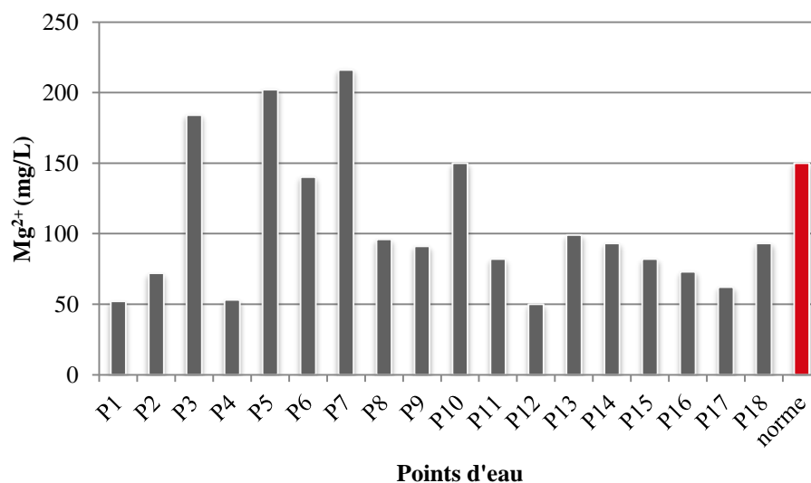
Figure III.4 : Variation de l'ion magnésium au niveau de la plaine de Sidi Bel Abbas
