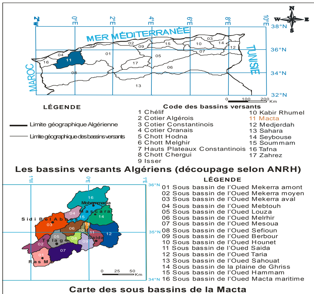
Figure. I.1 : Situation du bassin versant de la Macta(Otmane A, 2015)
