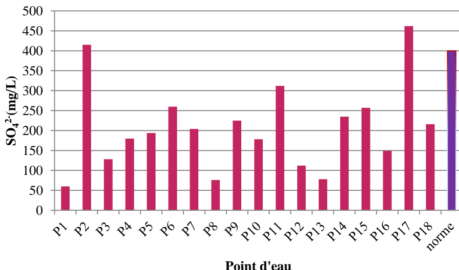
Figure III.9 :Variation des ions sulfates au niveau de la plaine de Sidi Bel Abbes
