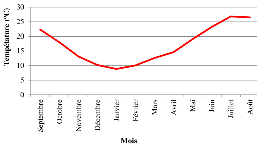
Figure II. 4 : Variation des températures moyennes mensuelles, à la station de Sidi Bel Abbès (1980/1981-2015/2016).
