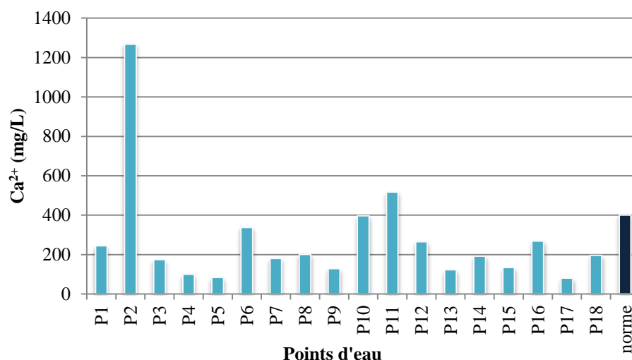
Figure III.3 : Variation de l'ion calcium au niveau de la plaine de Sidi Bel Abbas
