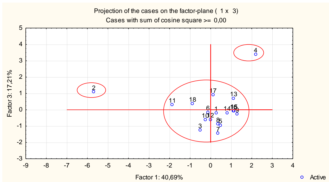
Figure IV.14 : Projection des individus (puits) sur le plan factoriel (F1 – F3)
