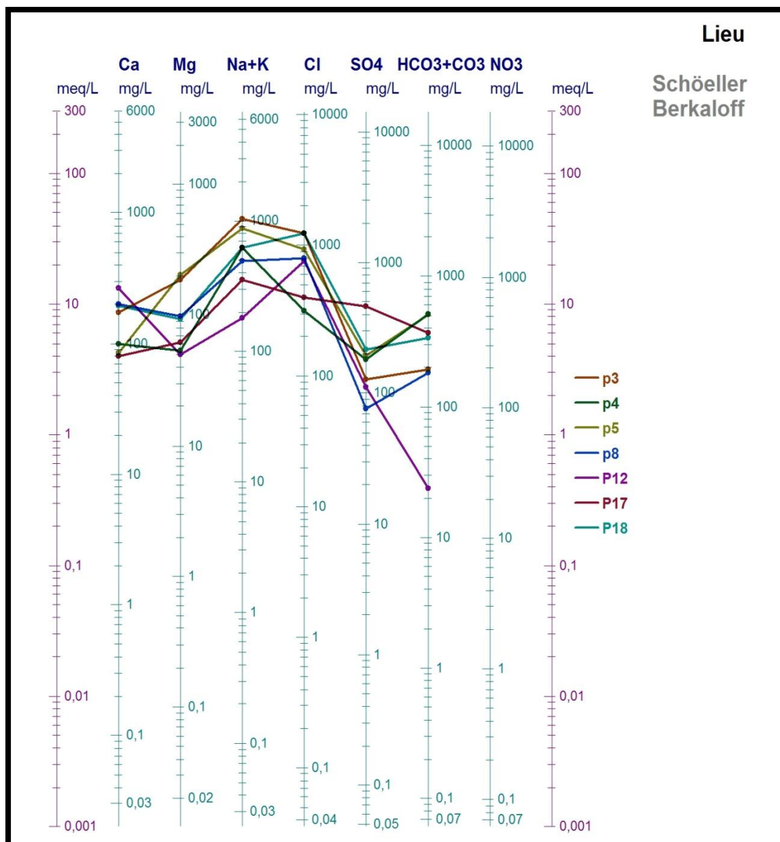
Figure III.10.b : Diagramme de Schöeller-Berkaloff (faciès chloruré sodique et potassique).
