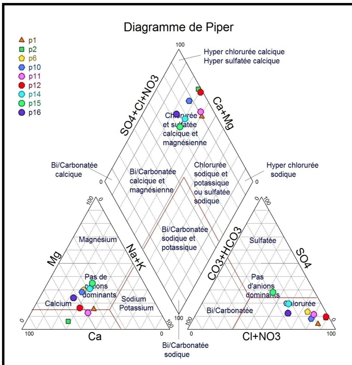
Figure III.11.a : Diagramme de Piper (faciès chloruré calcique).
