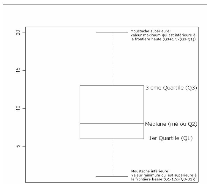
Figure IV.1 : Exemple de représentation d'un diagramme en boîte
