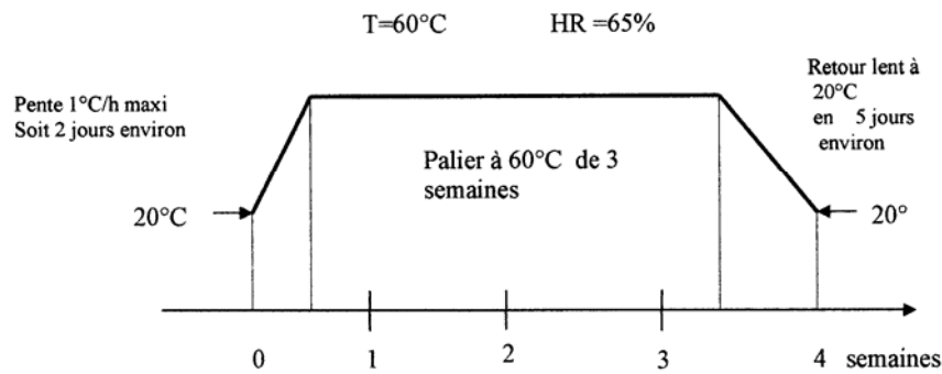
Figure 2. 9 Schéma du cycle de séchage en étuve programmable en T et HR [Dak, 2009]
