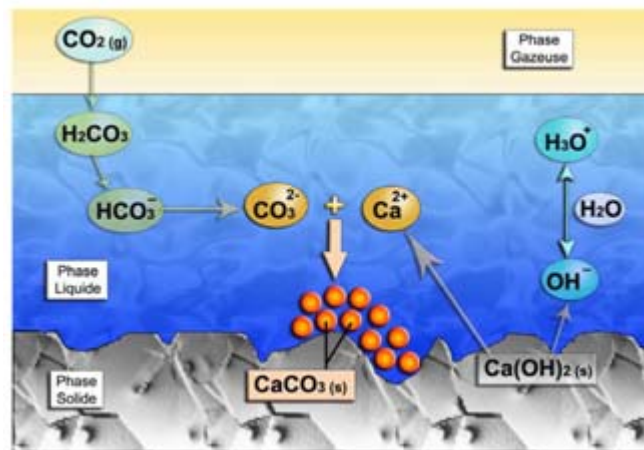
Figure 1. 11 Mécanisme de carbonatation de la portlandite [Thierry, 2005]
