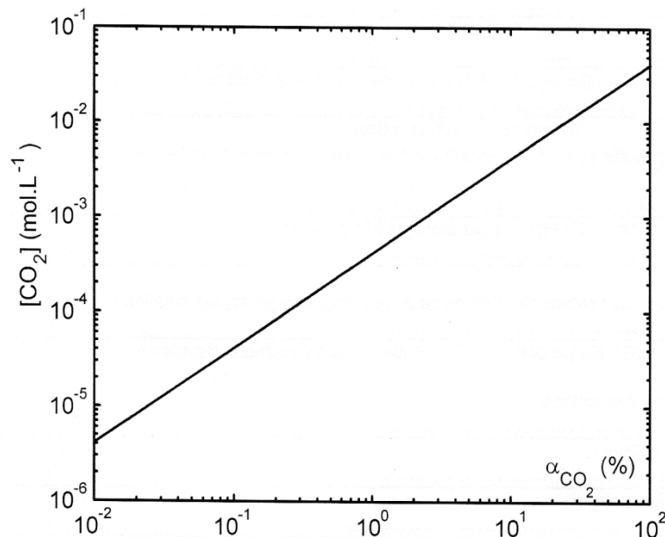
Figure 1. 1 Concentration en CO 2 dans la phase gazeuse en fonction de la fraction volumique \alpha_{CO_2} (à 20° C et sous une pression atmosphérique de 105 Pa) [Thiery, 2005]
