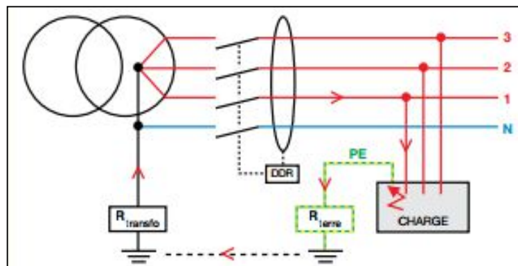
Figure 1: Dispositifs Différentiels Résiduels – DRR [1]
