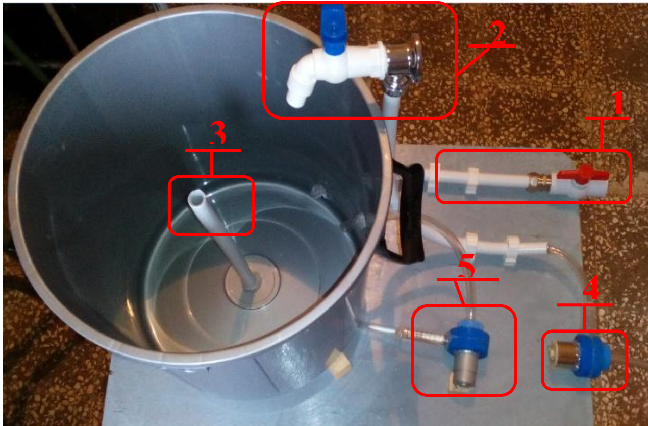
Figure.4.11 : vue de dessus de la maquette
