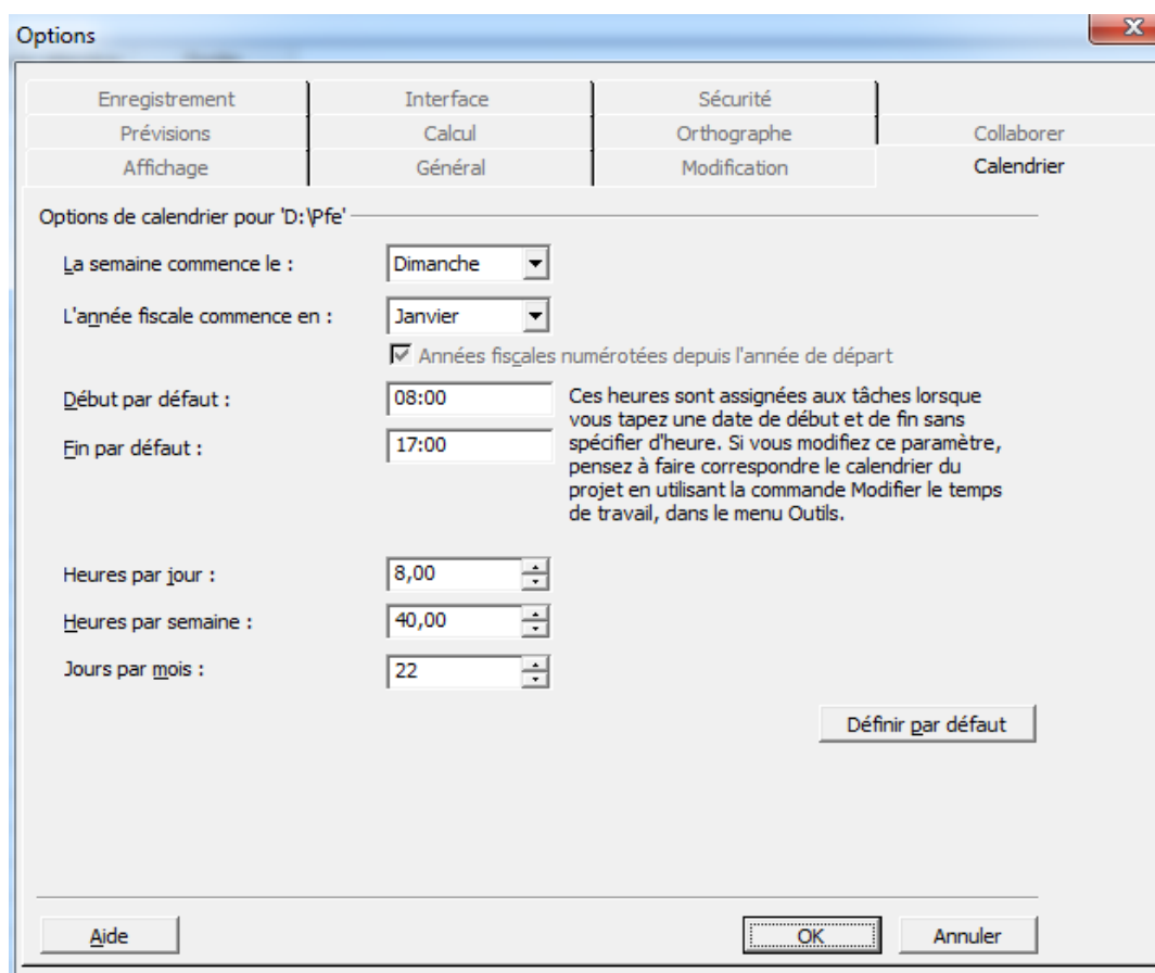
Figure 4. 3. Option calendrier sur MS Project
