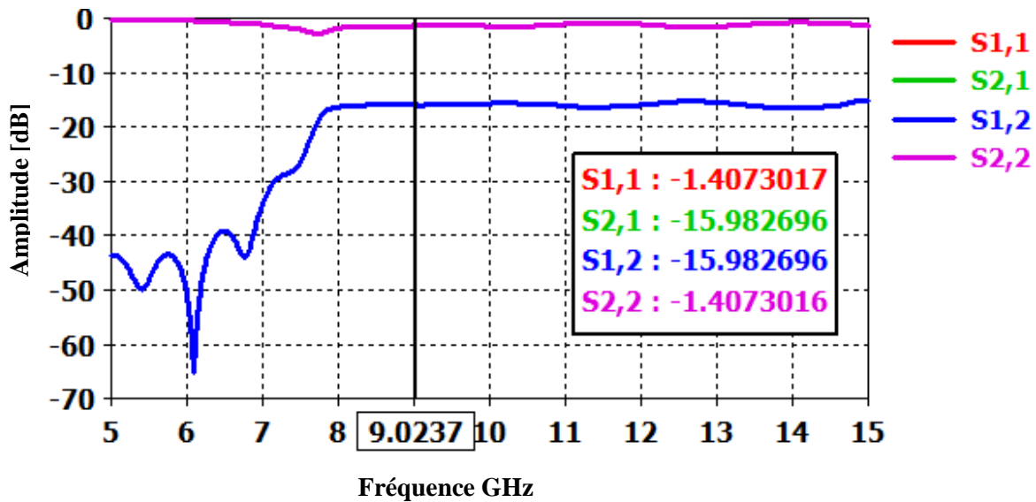
Figure III.4 : Résultat de simulation du guide SIW du coefficient de transmission et la puissance réfléchi. Les paramètres de guide sont définis par : d=2.3 mm, p=3.45 mm.
