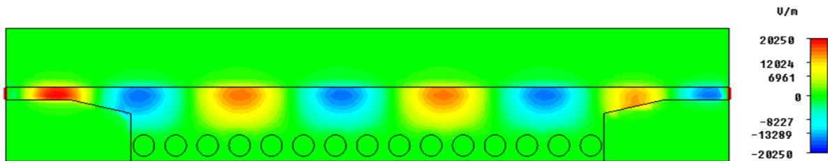
Figure III. 26 : Distribution du champ électrique dans le guide HMSIW.
