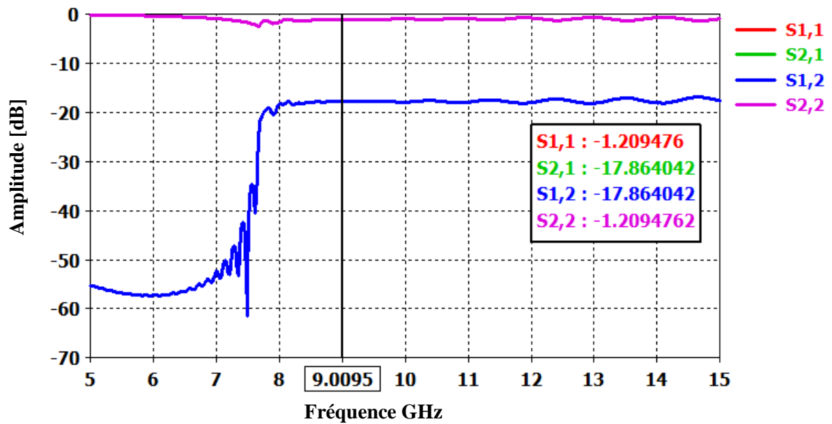
Figure III.9 : Résultat de simulation S1, 1 et S2, 1 pour 15 via-hôte et d=3.3 mm.
