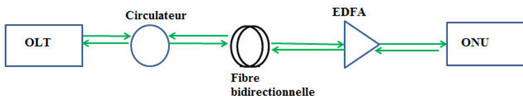
Figure 3.30 : La structure point à point dans OPTISYSTEM
