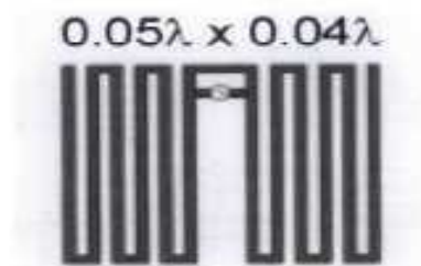
Figure 3.9 : Antenne de méandre- ligne equi-spaced ( f=953 MHz) avec l'alimentation de T-match [40].
