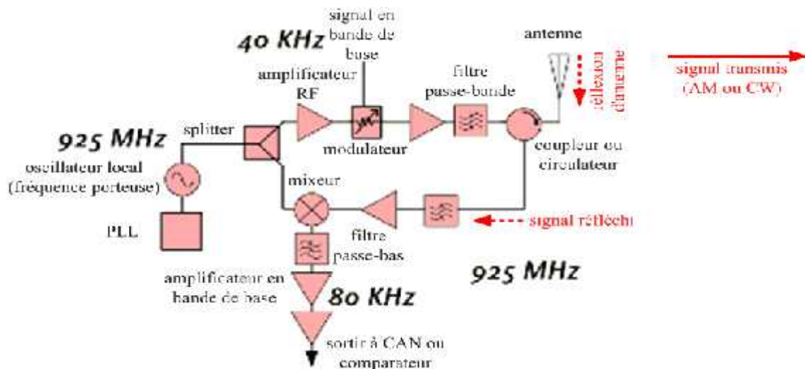
Figure 1.4 : Schéma synoptique fonctionnel d'un lecteur RFID (Front-end RF) [3].
