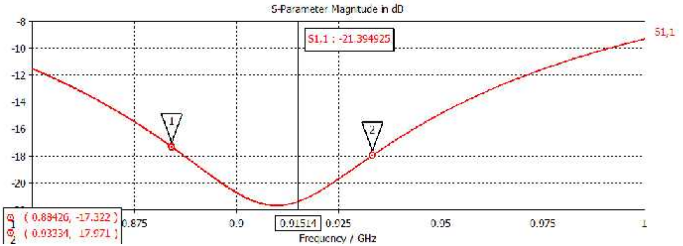
Figure 2.24 : tracé de S11 en fonction de fréquence.
