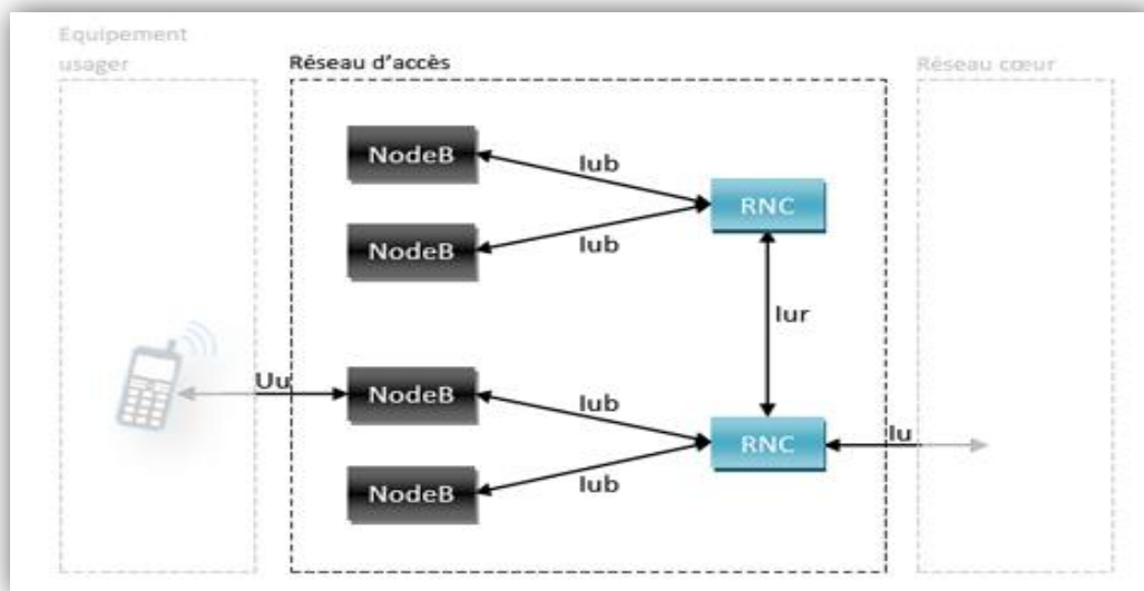
Figure II. 5: Architecture du réseau d'accès
