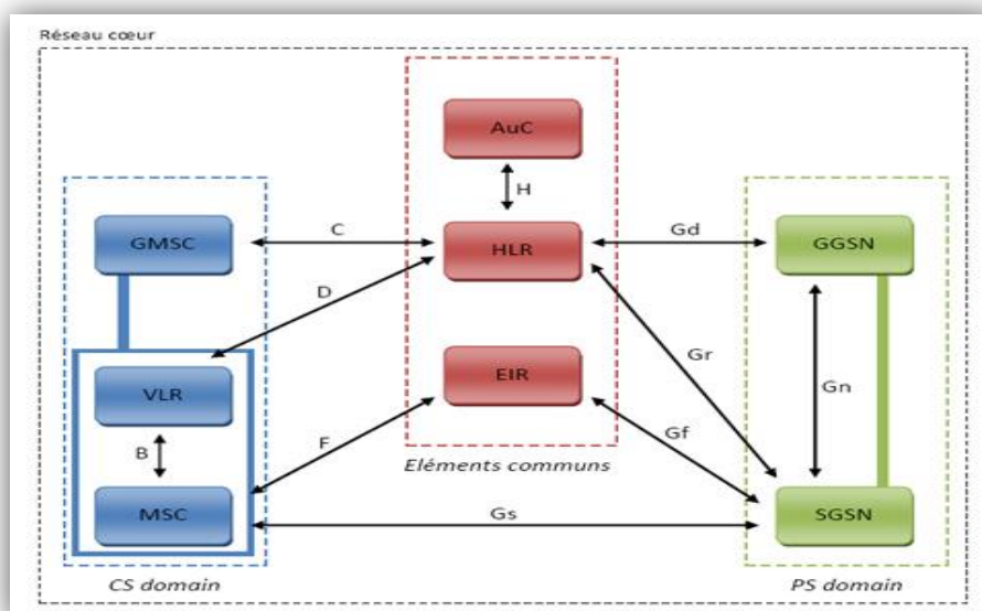
Figure II. 9: Architecture du réseau coeur (CN)
