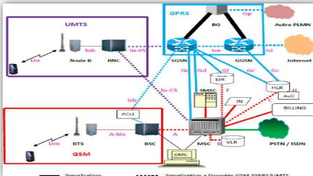
Figure II. 3: Vue générale des réseaux GSM, GPRS, UMTS
