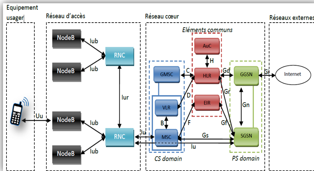
Figure II. 4: Architecture globale du réseau UMTS
