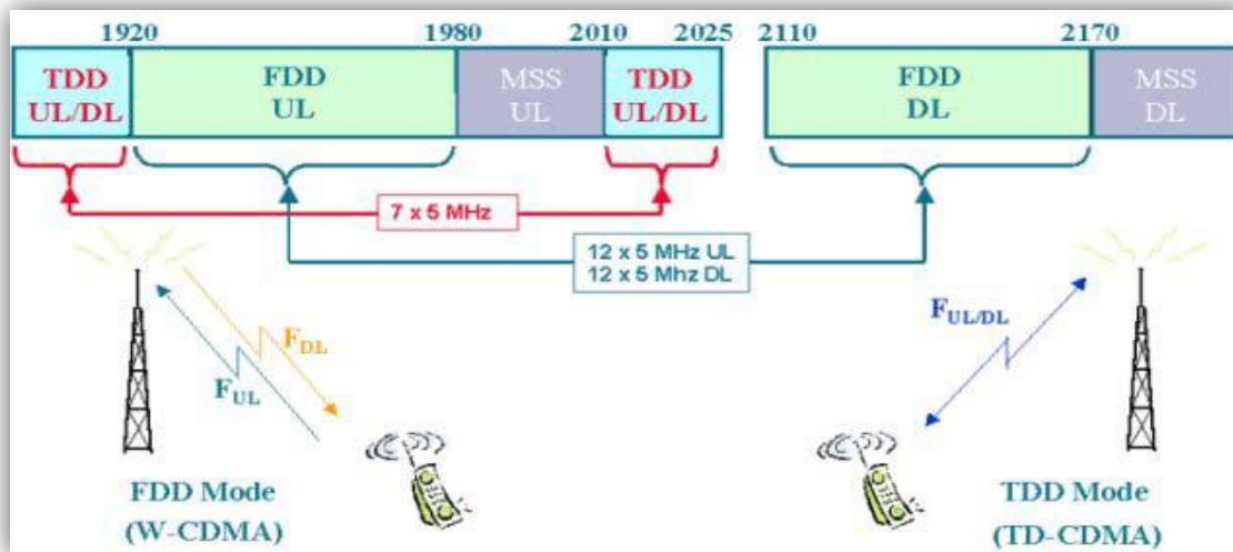
Figure II. 1: Allocation fréquentielle en UMTS
