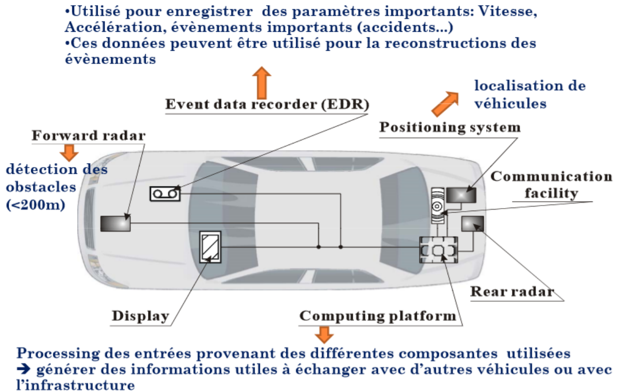
Figure I.3 : Les éléments constituant le véhicule intelligent [4].
