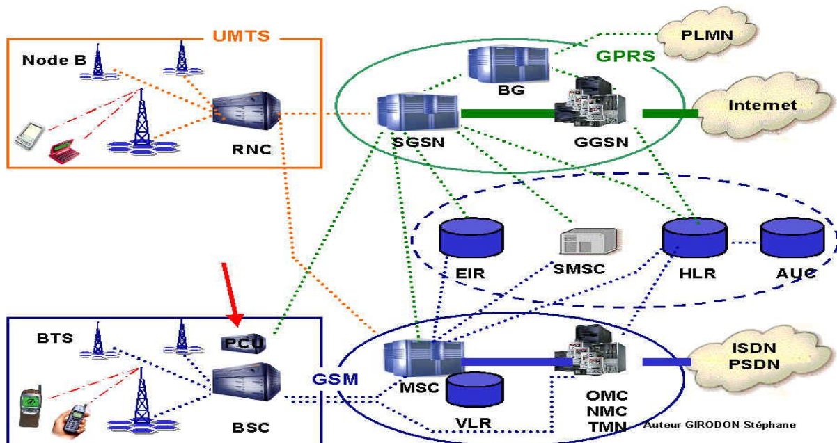
Figure I.5 : Architecture générale du réseau UMTS.
