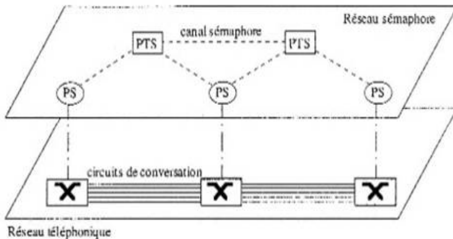
Figure I.10 : représentation fonctionnelle d'un réseau sémaphore.
