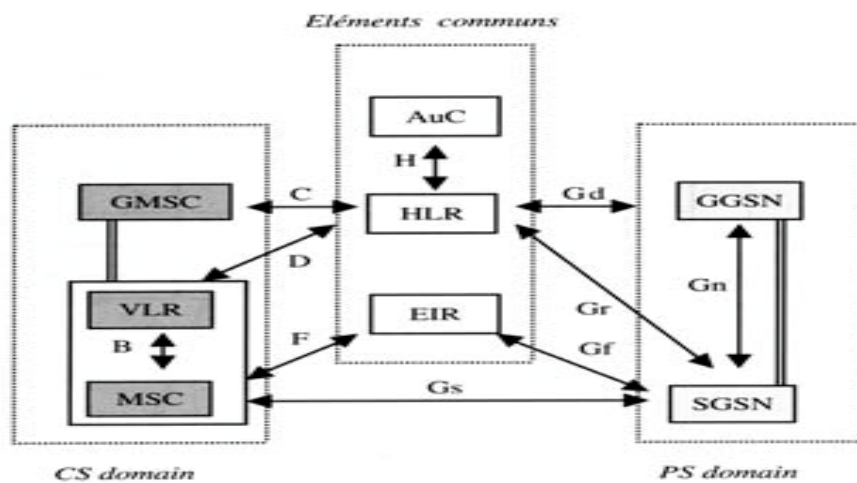
Figure I.6 : Le réseau cœur de l'UMTS.
