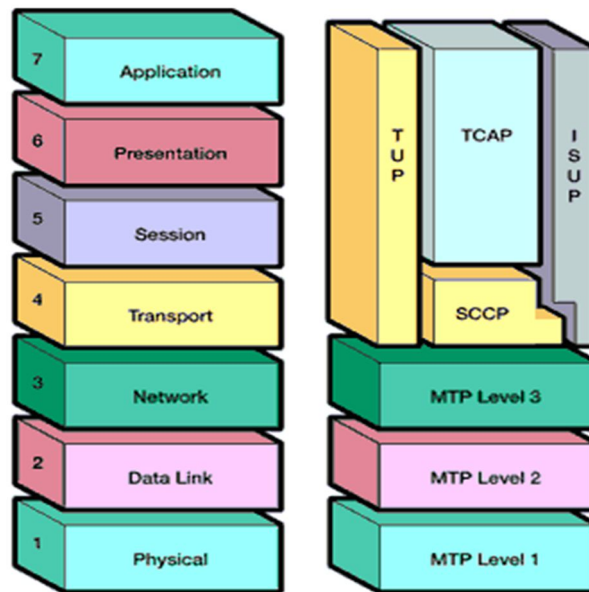
Figure I.11 : Le modèle de référence OSI et la pile de protocoles de communication SS7.
