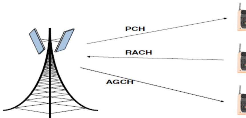
Figure I.8 : Les canaux de contrôles communs [].
