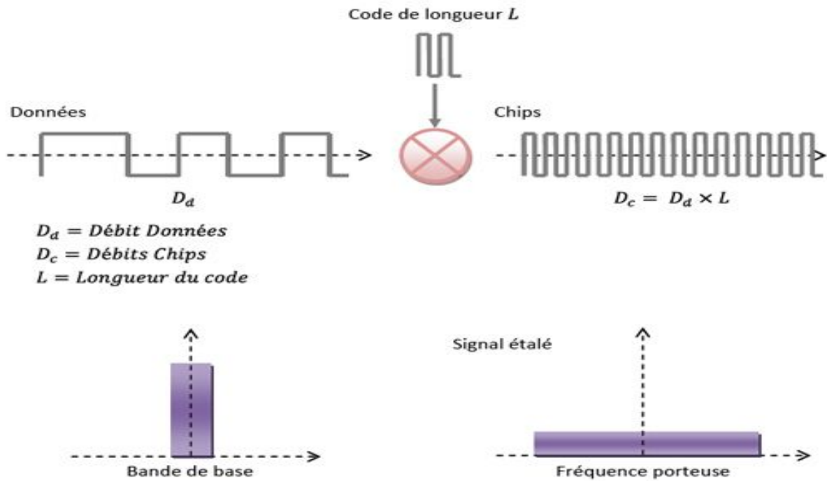
Figure I.4 : Principe de l'étalement de spectre.
