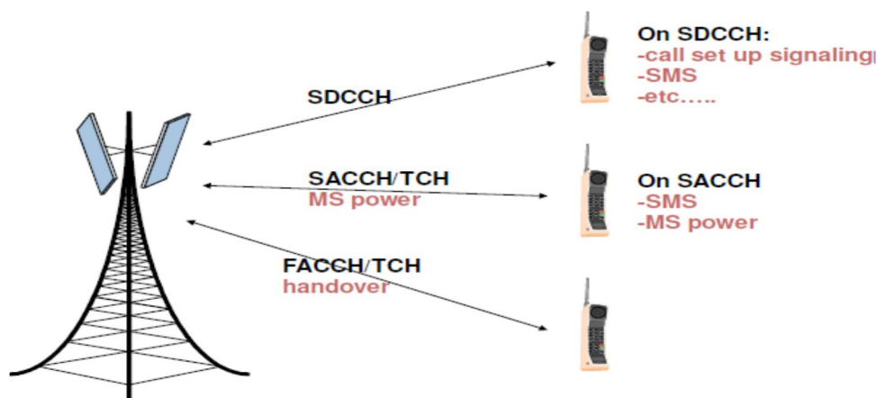
Figure I.9 : Les canaux de contrôle dédiés [1].
