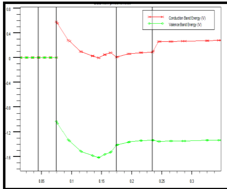
Figure III.3 : Diagramme de bandes d'énergie de MOS-PHEMT .
