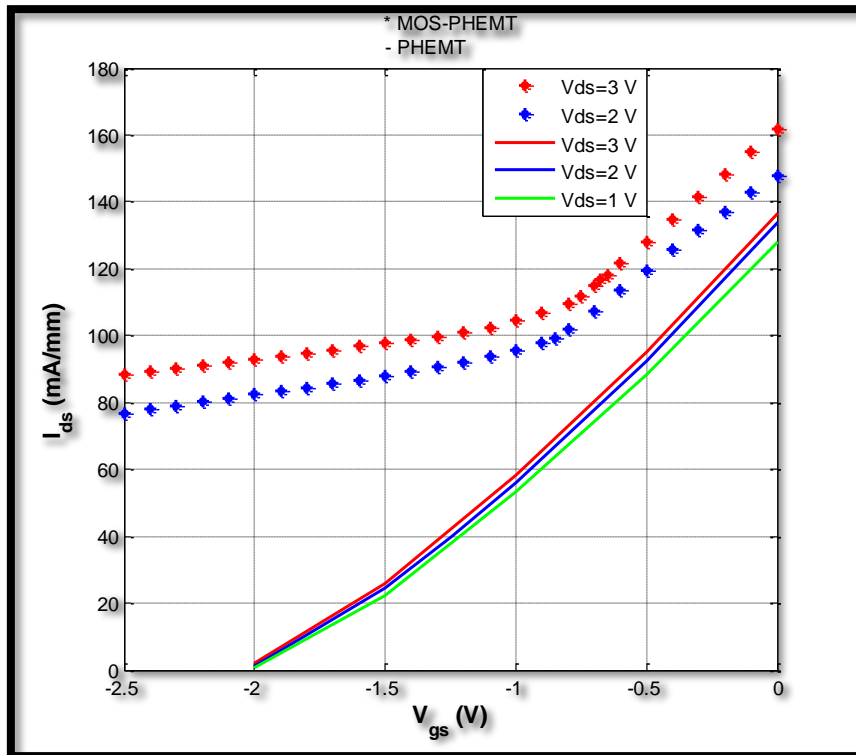
Figure III.11 : Comparaison entre les caractéristiques de transfert du MOS-PHEMT et du PHEMT
