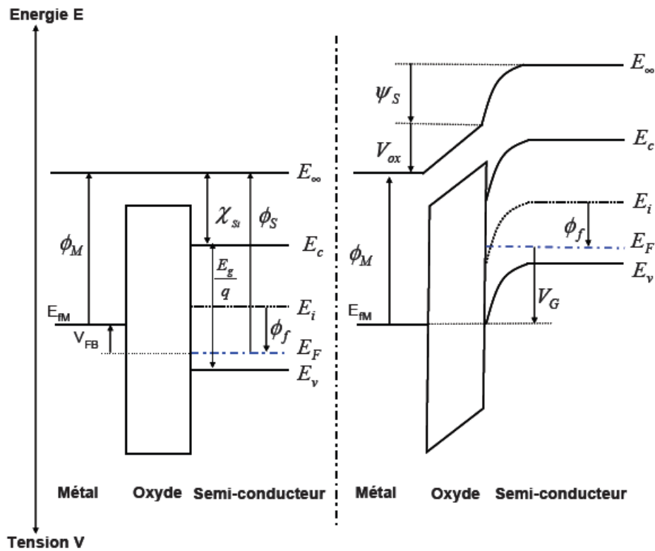
Figure II.1: Représentation schématique des bandes d'énergie d'un N-MOSFET, bandes plates (à gauche) et régime d'inversion faible (à droite).
