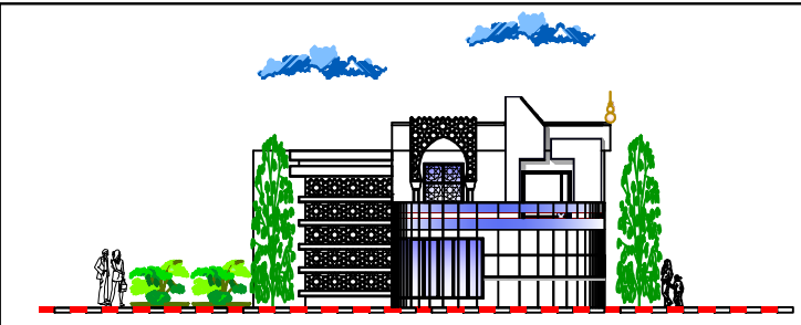
Façade Ouest
