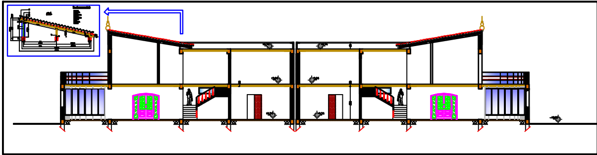
Coupe A-A
