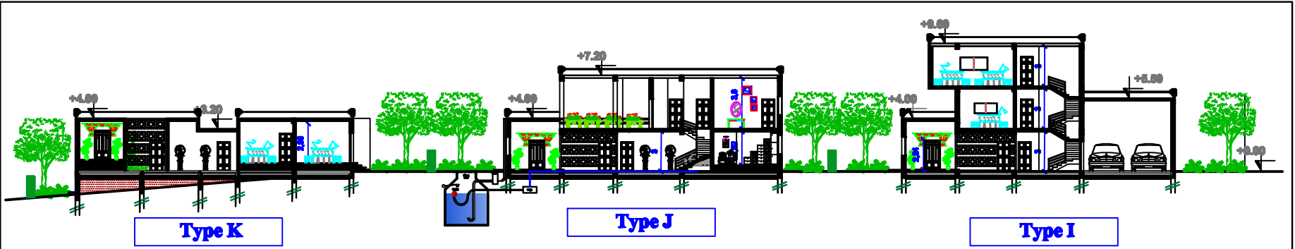
Coupe A-A
