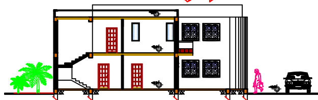
Coupe A-A
