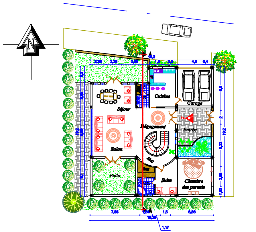
Plan RDC
