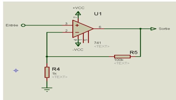
Figure 2.8 Amplificateur non-inverseur
