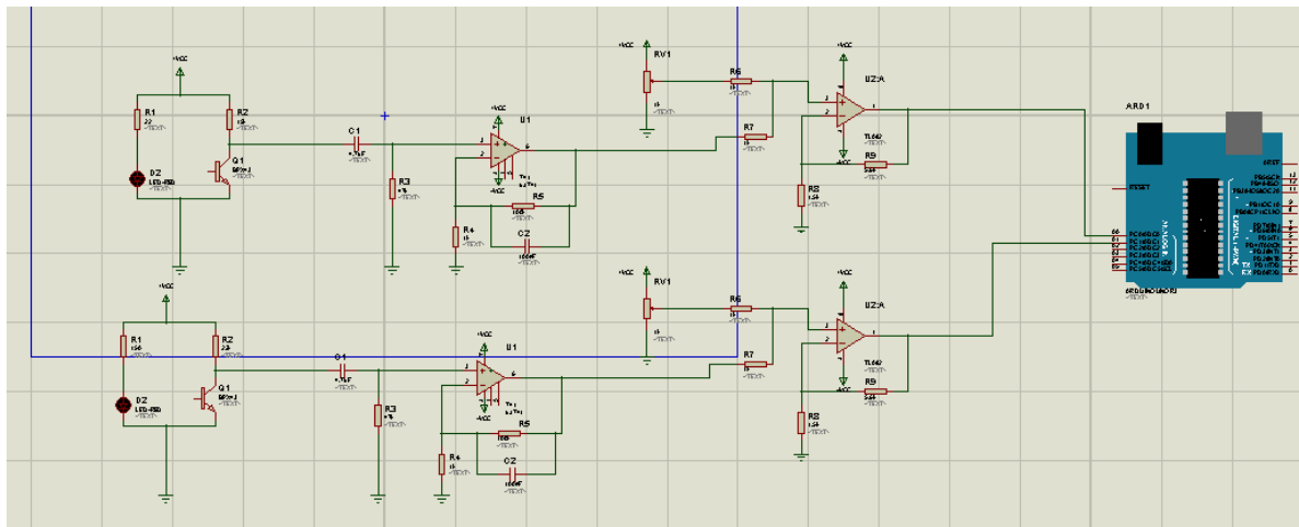
Schéma électrique de la carte
