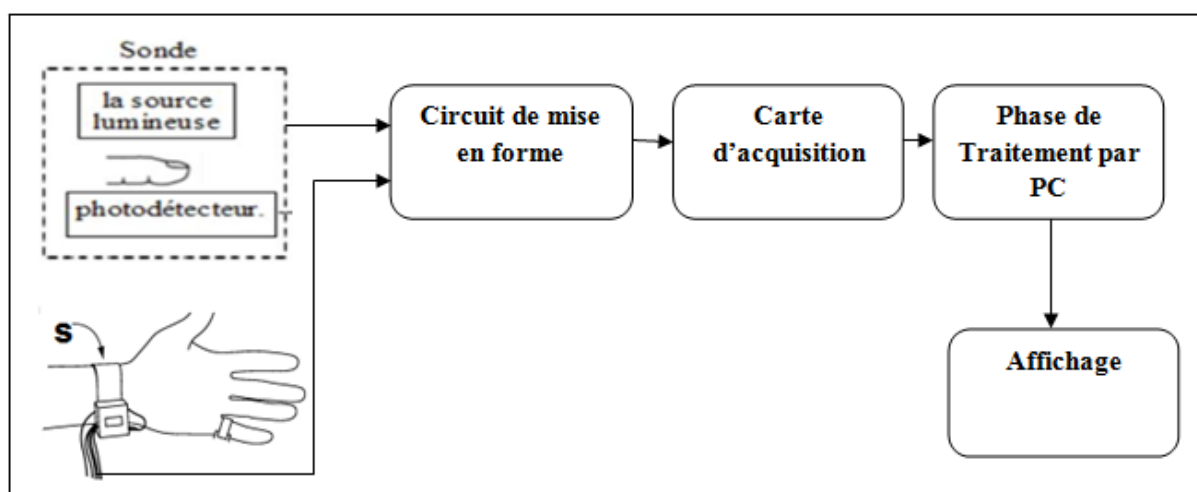
Figure 2.1 : schéma bloc
