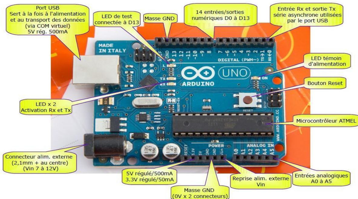
Figure3.1 Les différentes connexions d'une carte ArduinoUno [25]
