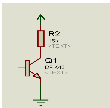
Figure 2.6 Circuit de détection
