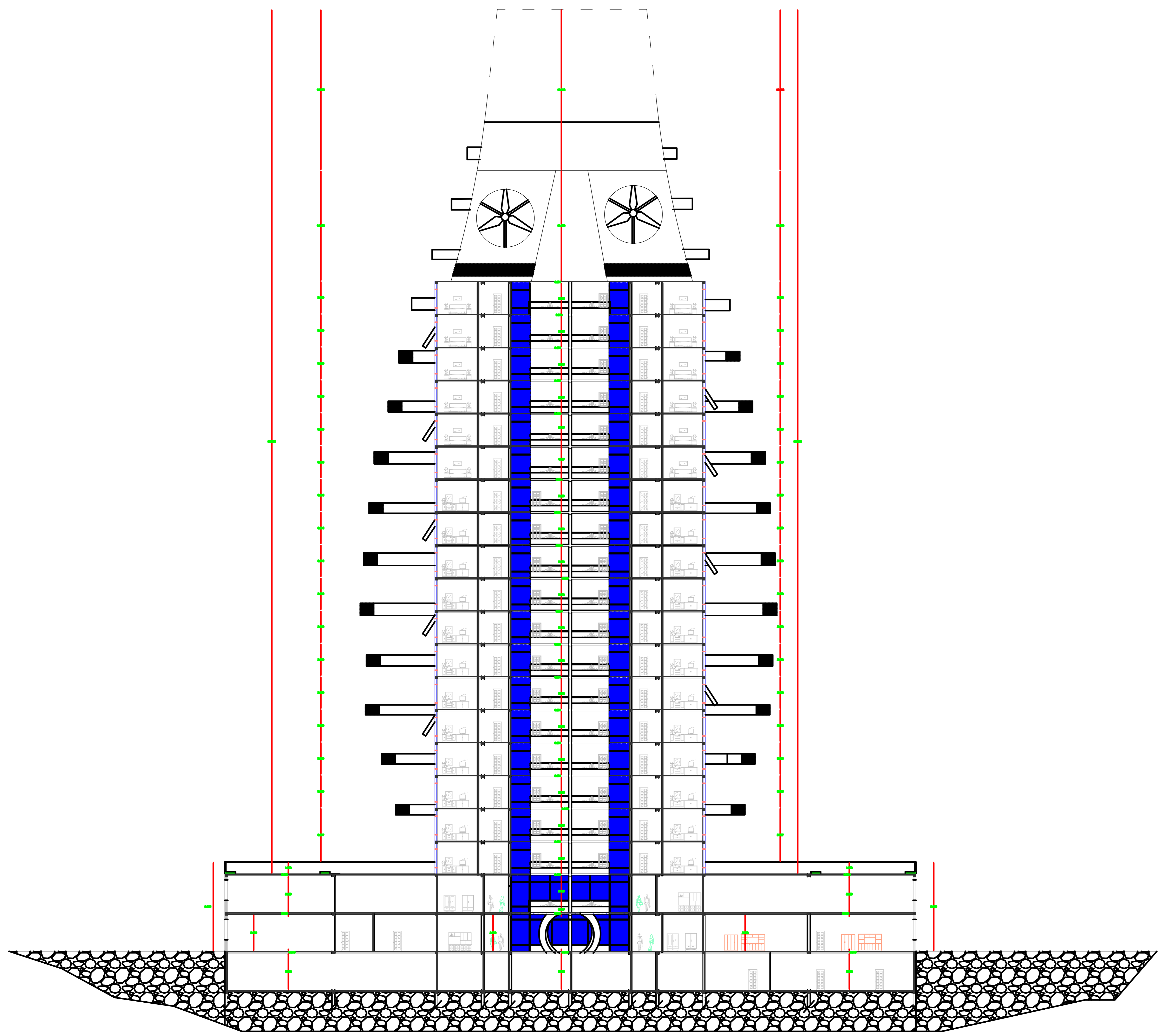
COUPE AA
