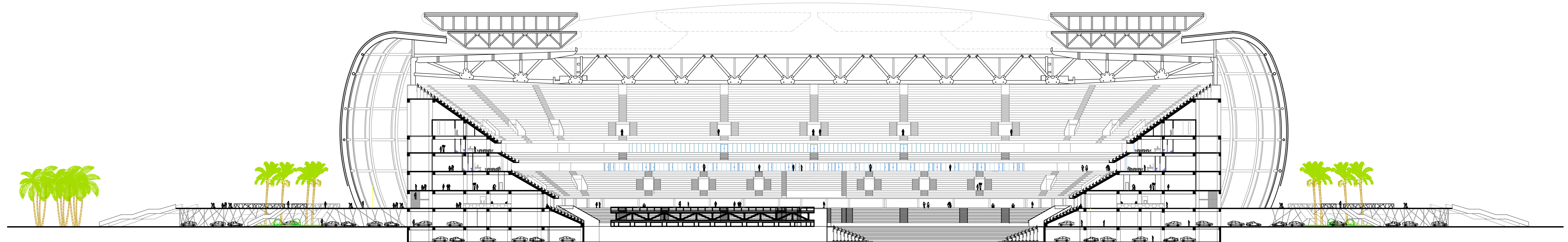
Coupe B-B
