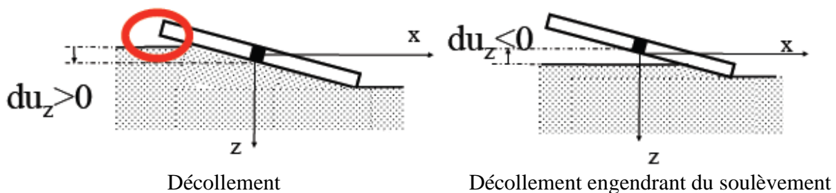
Figure 2.1 : phénomène de décollement et de soulèvement [Grange .S, 2008].
