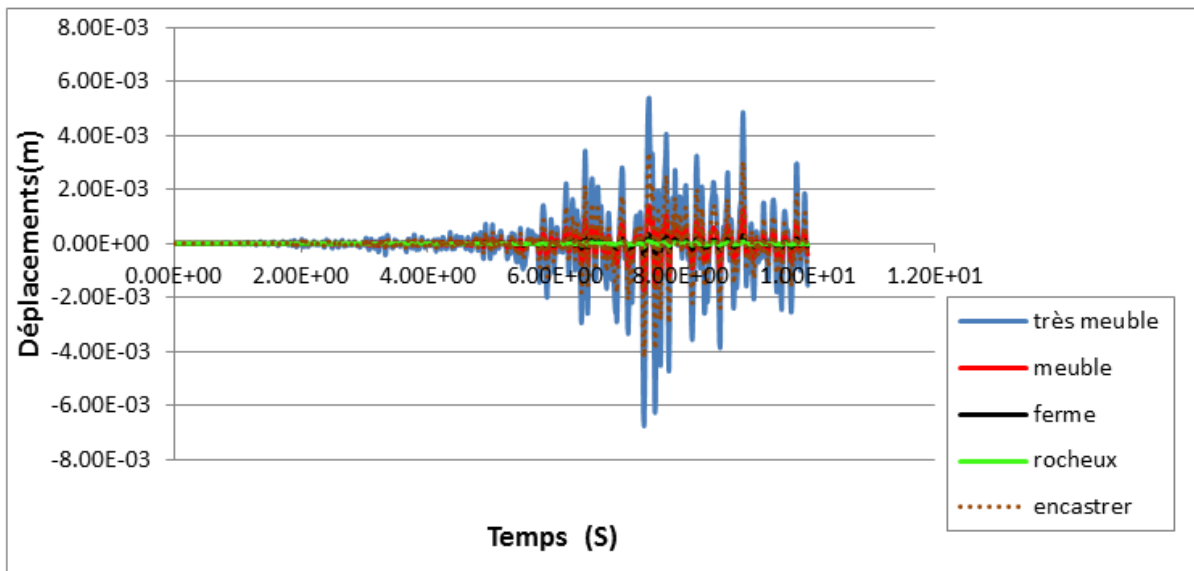
Figure 3.16 : Déplacement au sommet du poteau, séisme boumerdés (EF3D).
