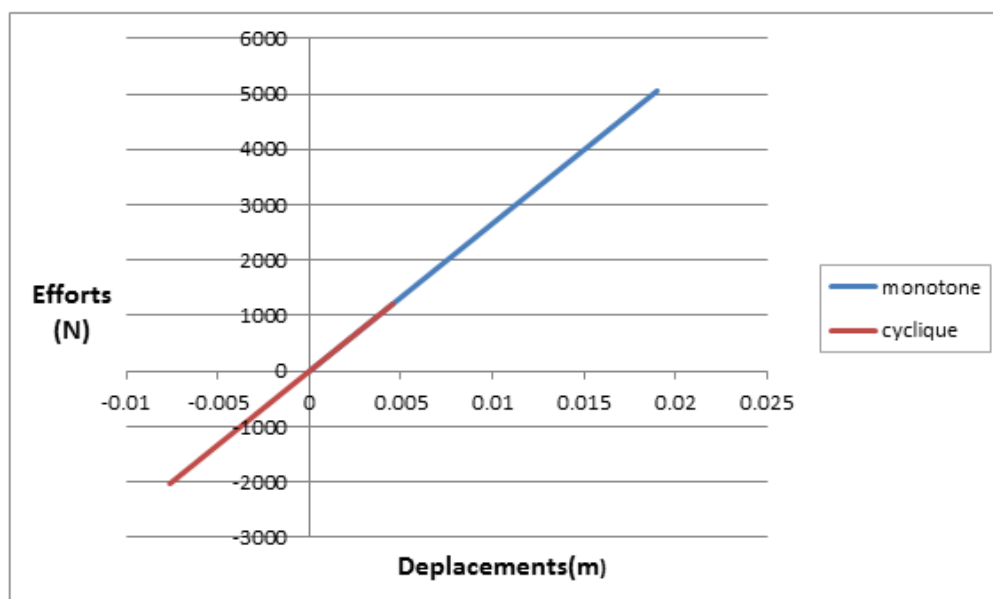
Figure 3.43 : Transitoire Vs. Push-Over pour le Modèle de Macro-élément (S3).
