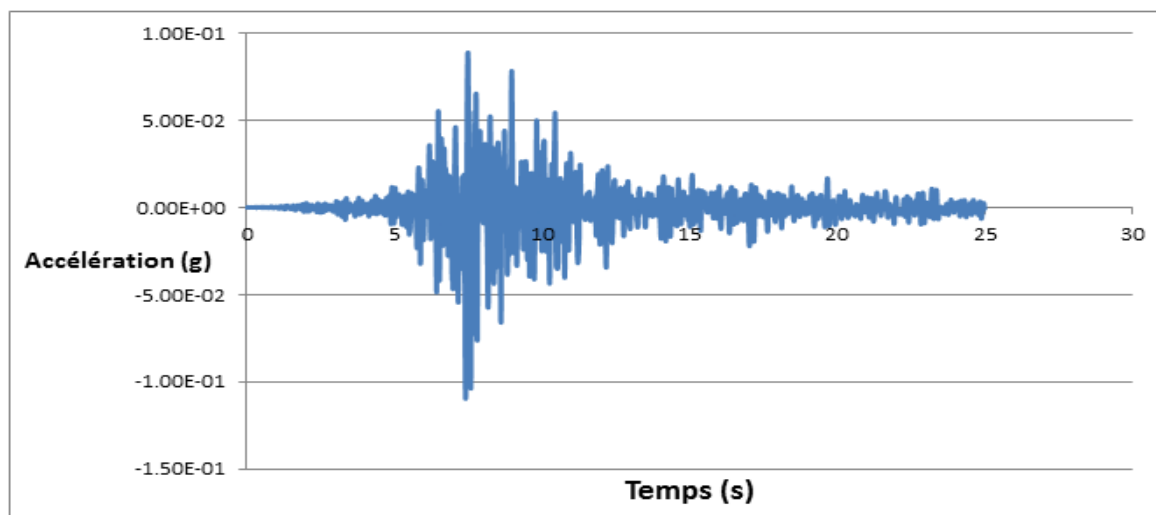
Figure 3.4 : Accélérogramme de Boumerdes.
