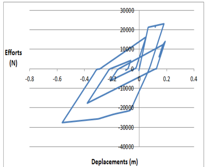
Figure 3.35: Force-déplacement Modèle de Macro-élément (S2)
