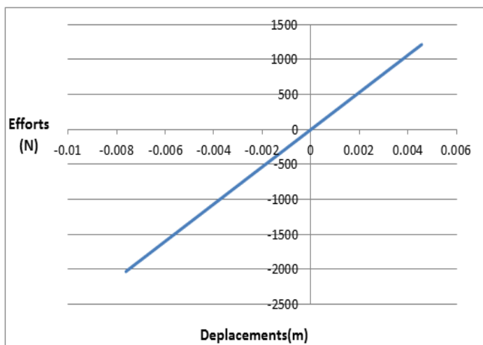
Figure 3.27 : Force-déplacement Macro-élément (S3)
