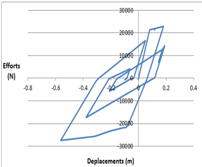
Figure 3.36 : Force-déplacement Modèle de Macro-élément (S3)
