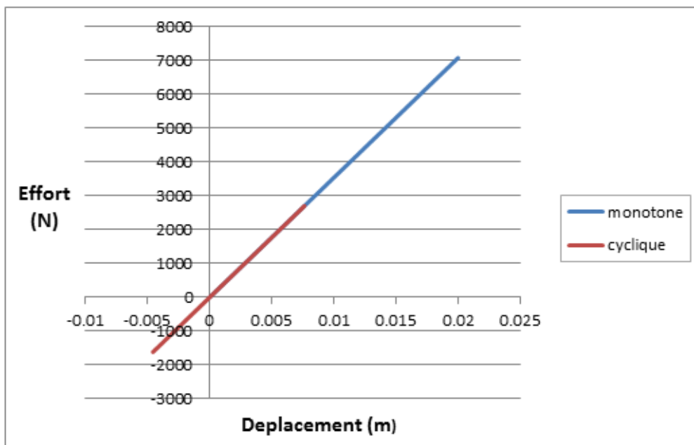
Figure 3.38 : Transitoire Vs. PushOver pour le Modèle Eléments Finis3D (S1).
