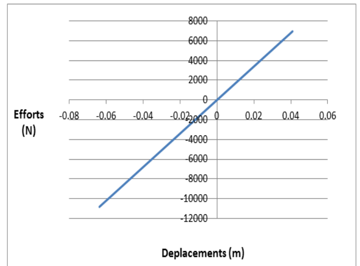
Figure 4.17 : Force-déplacement Modèle Eléments Finis 3D (S4)
