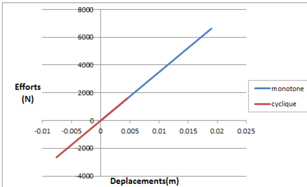
Figure 3.41 : Transitoire Vs. Push-Over pour le Modèle de Macro-élément (S1).
