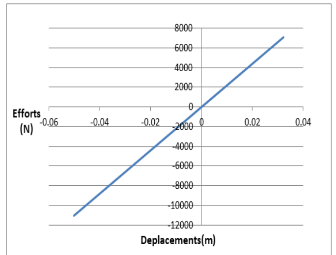
Figure 4.15 : Force-déplacement Modèle Eléments Finis 3D (S2)
