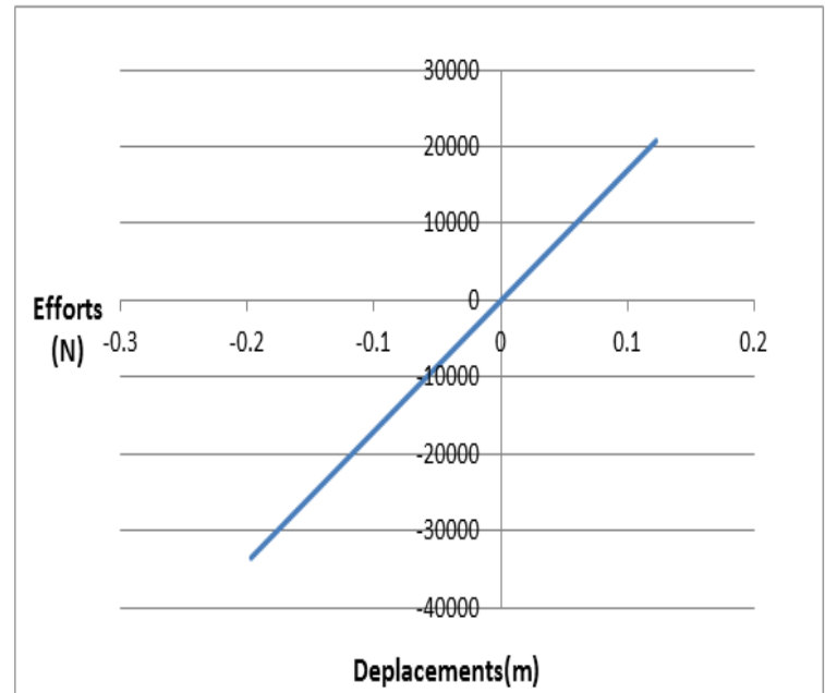
Figure 4.26 : Force-déplacement Modèle Eléments Finis 3D (S4)
