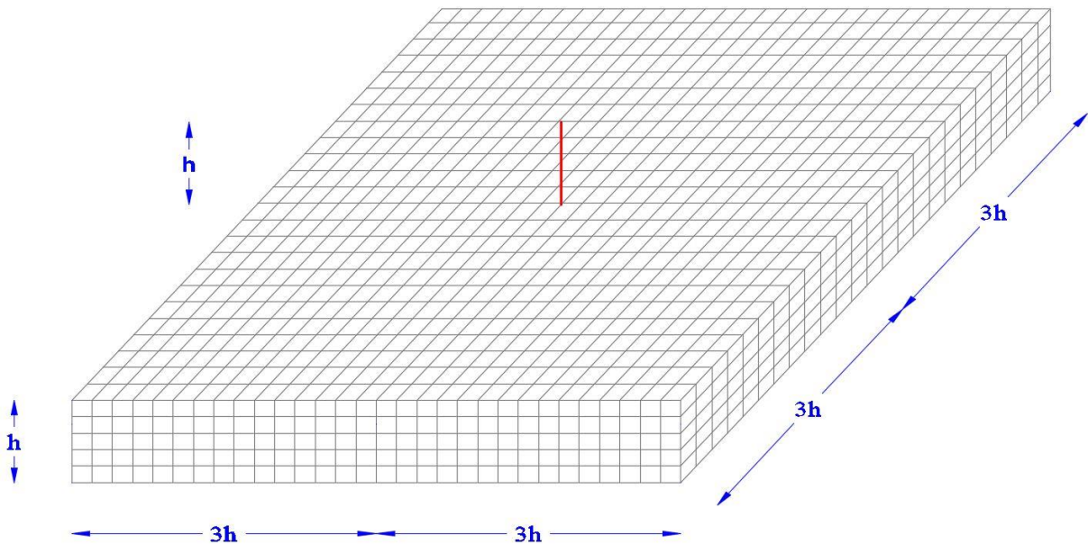
Figure 3.7 : Modèle en éléments finis sol-structure.
