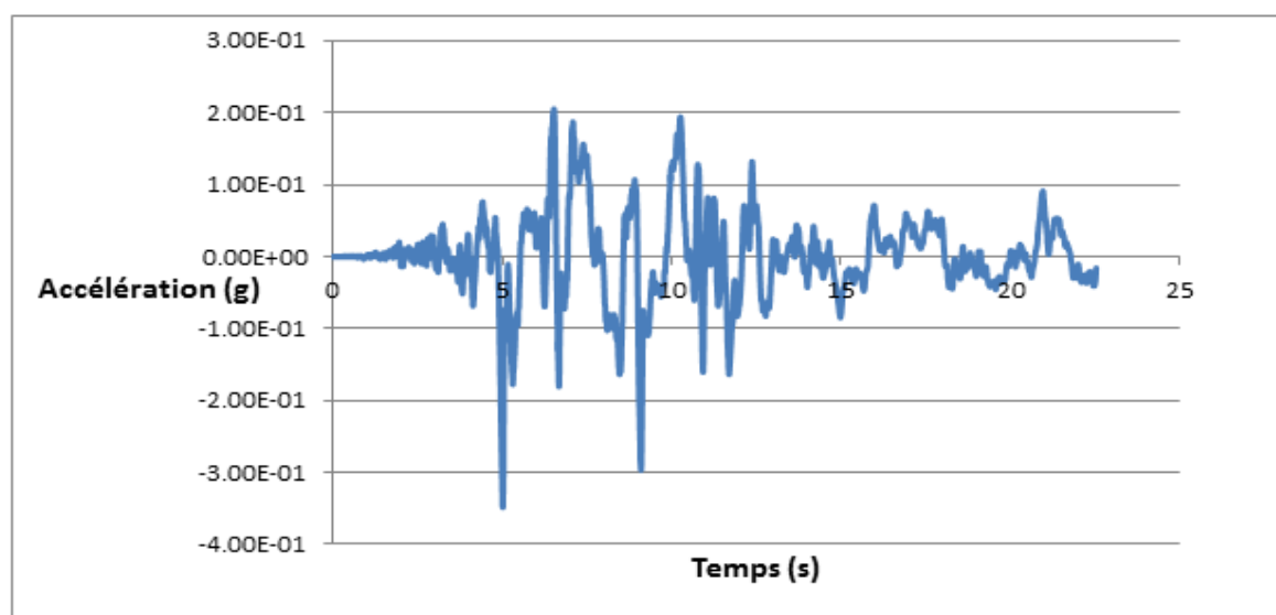
Figure 3.5 : Accélérogramme de Kocaeli.
