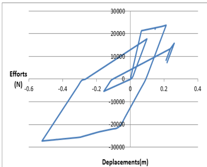
Figure 3.31 : Force-déplacement Modèle Eléments Finis (S3)
