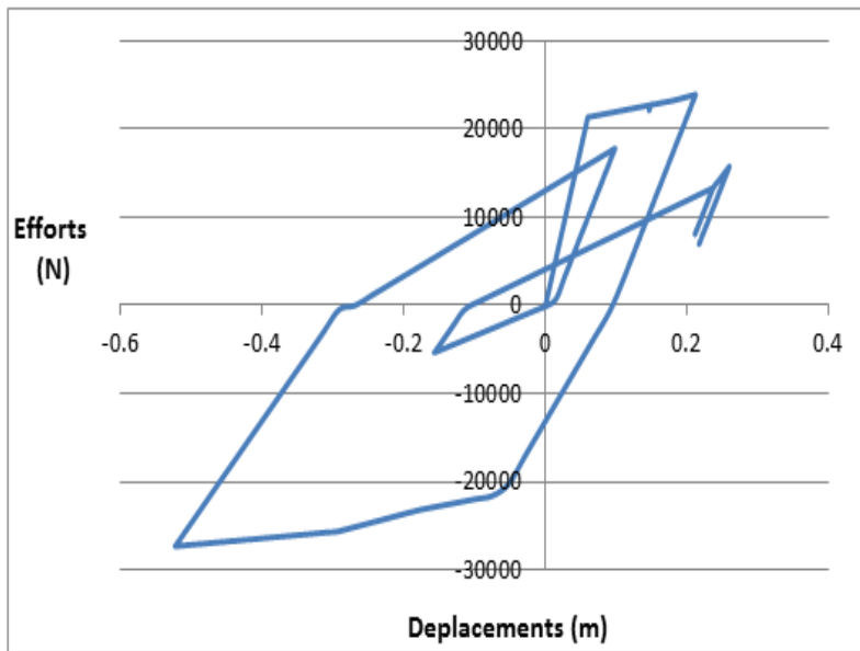
Figure 3.33 : Force-déplacement encastré
