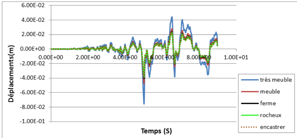
Figure 4.7 : Déplacement au sommet de la structure, séisme Kocaeli (Macro-élément).
