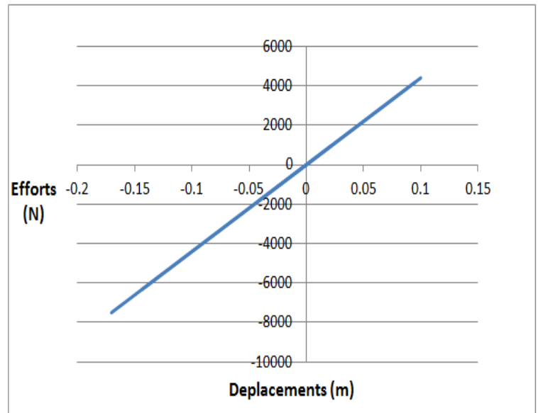
Figure 4.28 : Force-déplacement Modèle de Macro-élément (S2)
