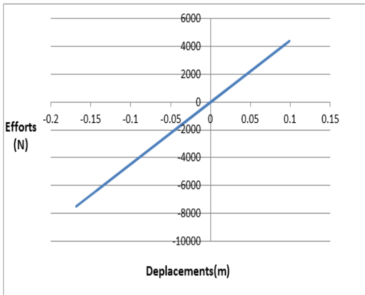
Figure 4.27 : Force-déplacement Modèle de Macro-élément (S1)
