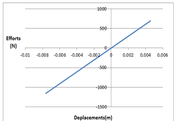
Figure 3.28 : Force-déplacement Macro-élément (S4)
