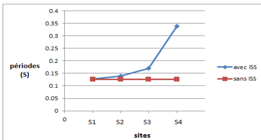
Figure 3.8 : Evaluation des périodes fondamentales pour différents sites, Poteau (Model EF3D).
