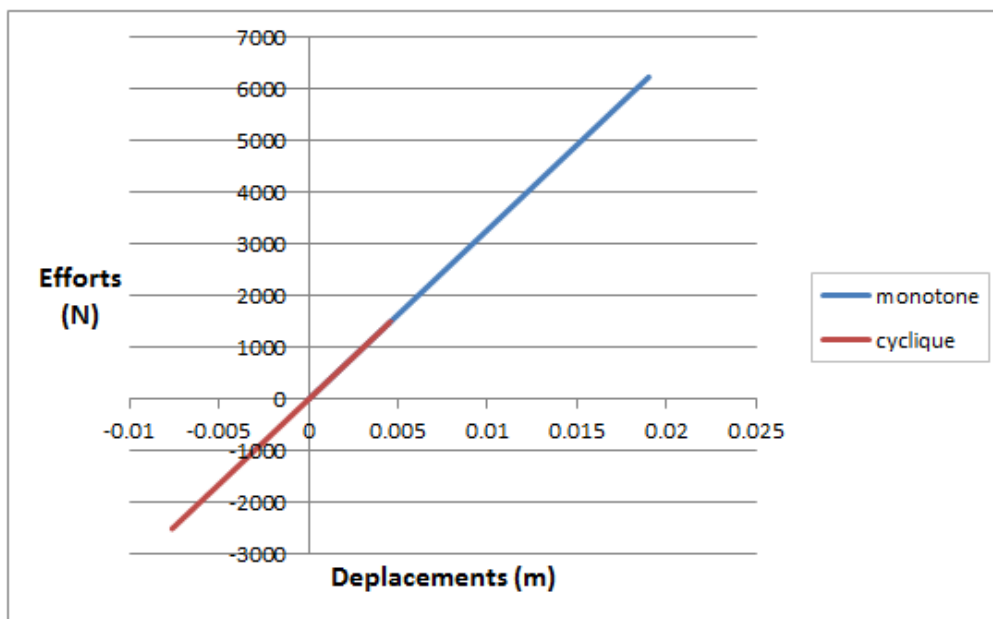
Figure 3.42 : Transitoire Vs. Push-Over pour le Modèle de Macro-élément (S2)
