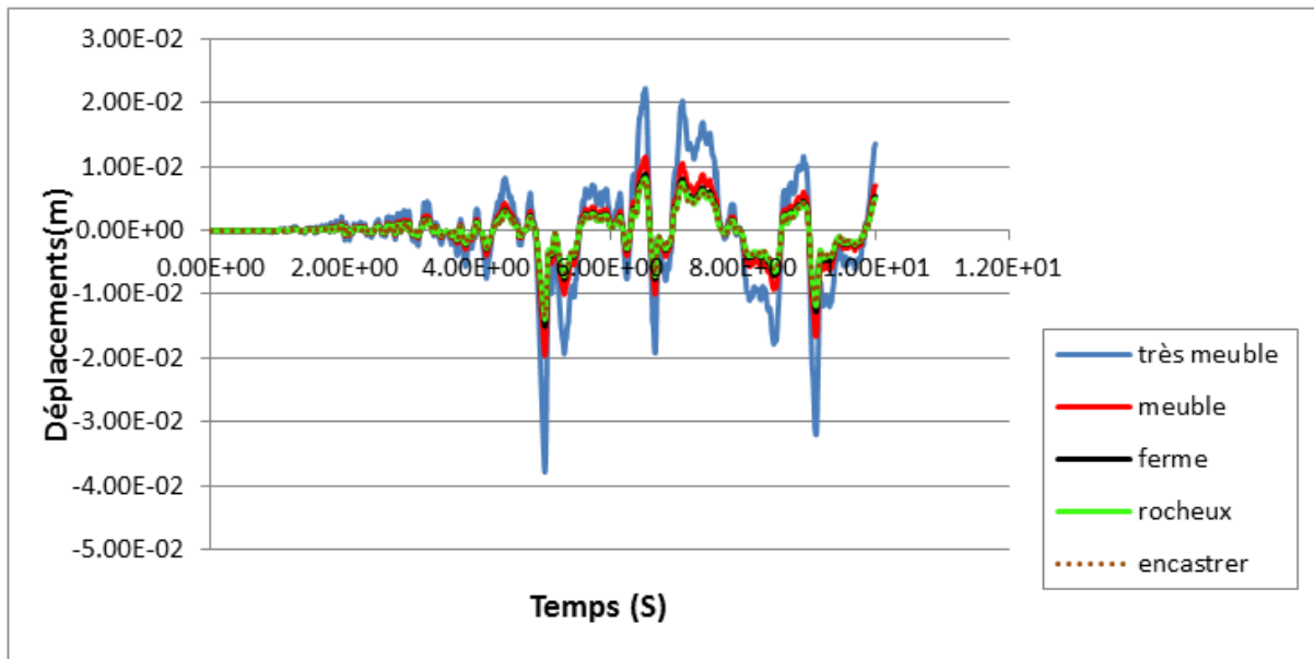
Figure 3.19 : Déplacement au sommet du poteau, séisme Kocaeli (Macro-élément).
