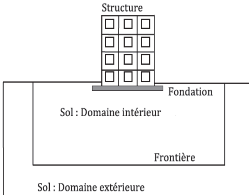
Figure1.5 : Méthode de réduction de domaine [Seghir A., 2011].
