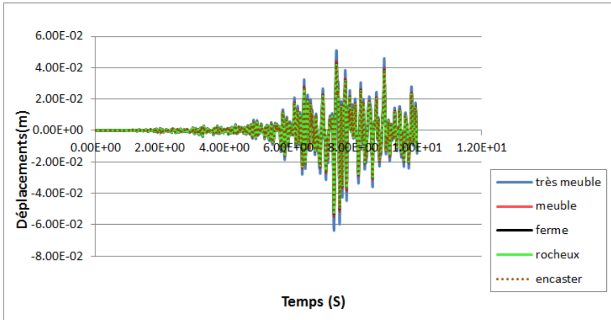
Figure 4.11 : Déplacement au sommet de la structure, séisme boumerdés (Macro-élément).
