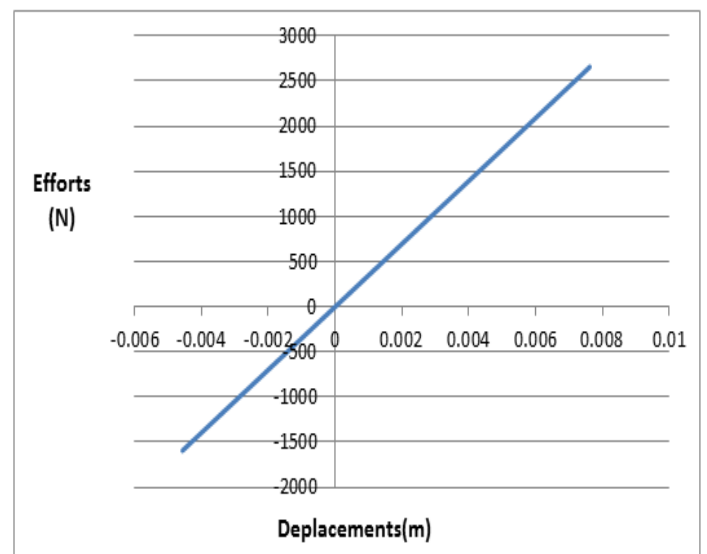
Figure 3.21 : Force-déplacement Eléments Finis 3D (S2)
