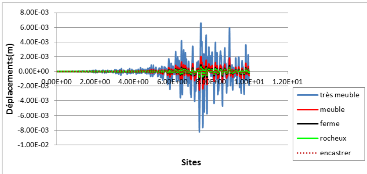
Figure 3.11 : Déplacement au sommet du poteau séisme boumerdés (Macro-élément).
