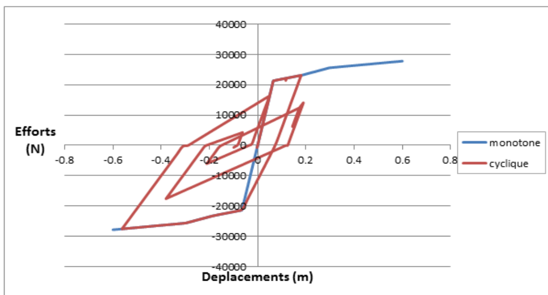
Figure 3.50 : Transitoire Vs. Push-Over pour le Modèle de Macro-élément (S2).
