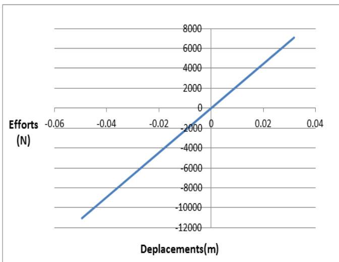
Figure 4.14 : Force-déplacement Modèle Eléments Finis 3D (S1)
