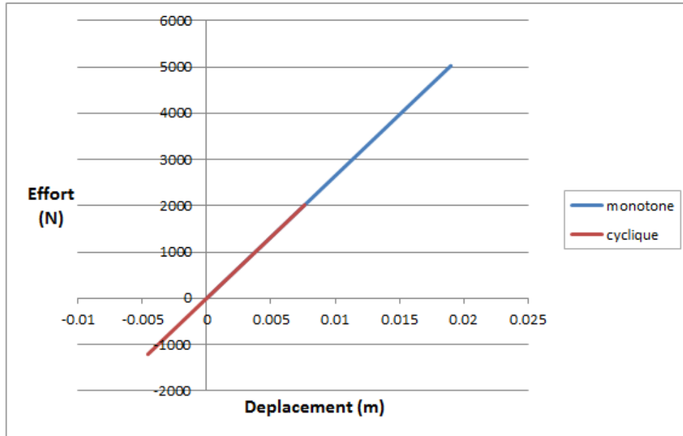
Figure 3.40 : Transitoire Vs. Push-Over pour le Modèle Eléments Finis3D (S1).
