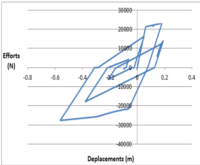
Figure 3.34 : Force-déplacement Modèle de Macro-élément (S1)
