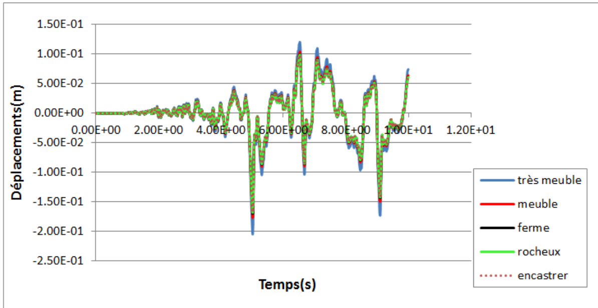
Figure 4.13 : Déplacement au sommet de la structure, séisme Kocaeli (Macro-élément).
