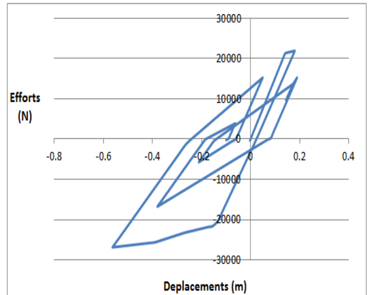
Figure 3.37 : Force-déplacement Modèle de Macro-élément (S4)
