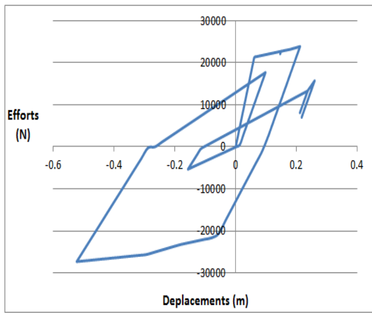
Figure 3.30 : Force-déplacement Modèle Eléments Finis (S2)
