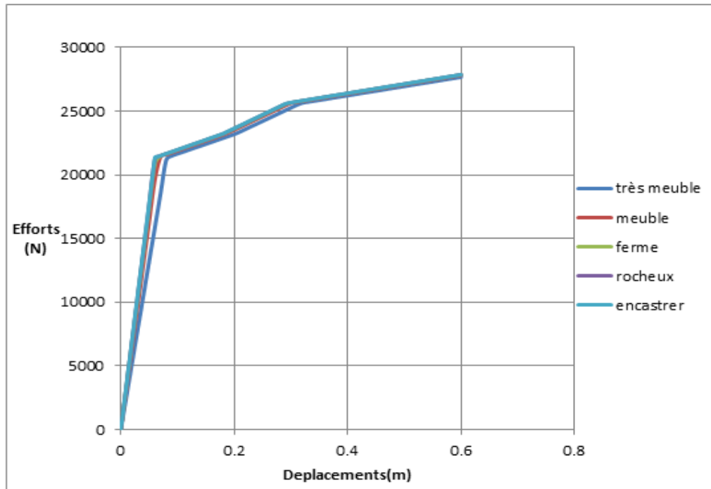
Figure 3.14 : Effort-déplacements pour différent sites avec l'encastrement (Modèle EF3D)
