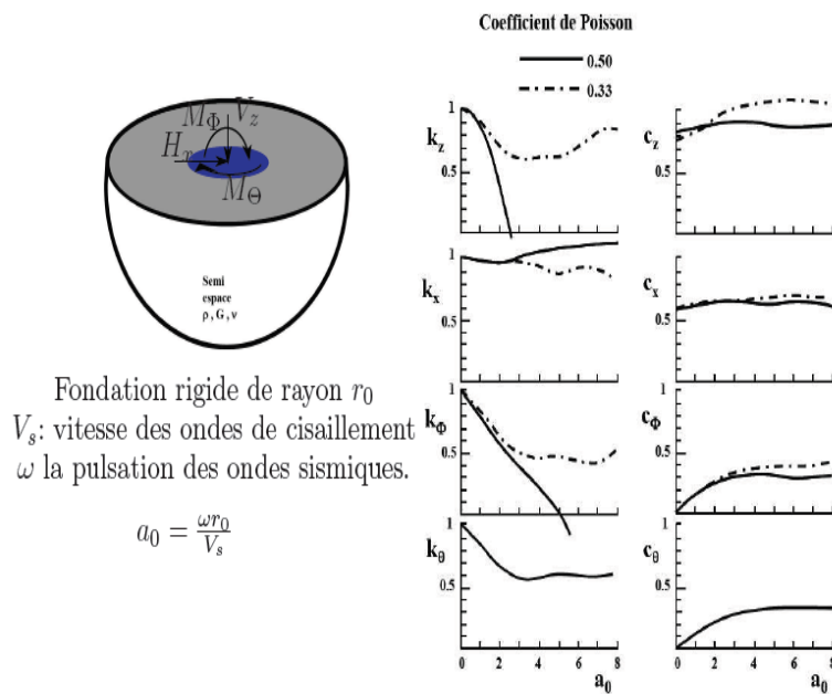
Figure 1.13: Termes d'impédance (raideur et amortissement) pour une fondation superficielle circulaire selon Pecker [Pecker A., 1984].
