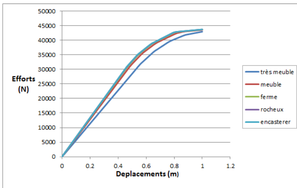
Figure 4.8 : Effort-déplacements pour différent sites (Modèle Eléments Finis):
