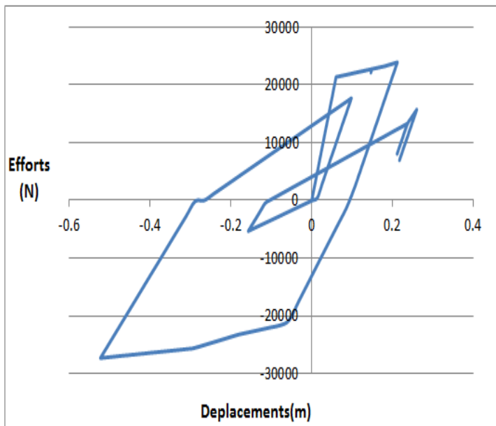
Figure 3.29 : Force-déplacement Modèle Eléments Finis (S1)
