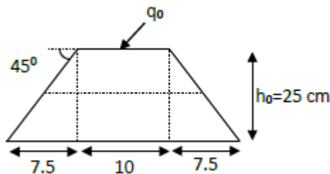
Figure IV.7 : Chargement appliqué
