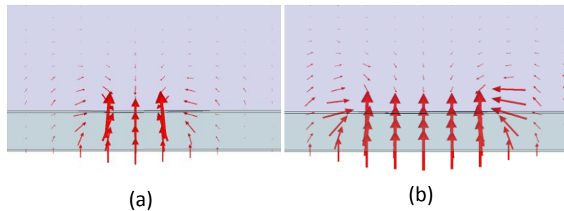
Figure I.16. La distribution de champ électrique E . (a) à l'entrée et (b) à la sortie de la transition entre la ligne micro-ruban et le guide GIS [60].
