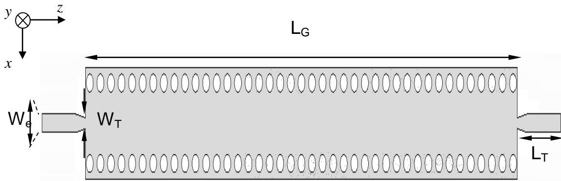
Figure III. 19. Structure du guide GIS opérant en bande Ka. Les paramètres du guide sont donnés par: a_s=4.36\text{ mm} , d=0.967\text{ mm} , s=1.45\text{ mm} , W_e=1.47\text{ mm} , W_T=0.48\text{ mm} , L_T=9.91\text{ mm} , L_G=60\text{ mm} .
